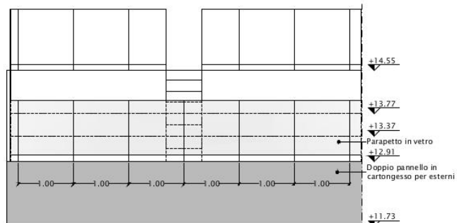
PROSPETTO FRONTALE Scala 1:50
